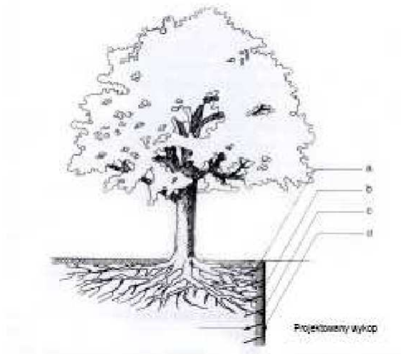
Rys. 6. Przykład wykonania ekranu korzeniowego: a. bryła korzeniowa, b. ziemia urodzajna, c. folia, d. szalunek, e. kotwy utrzymujące ekran (źródło: jak wyżej)
