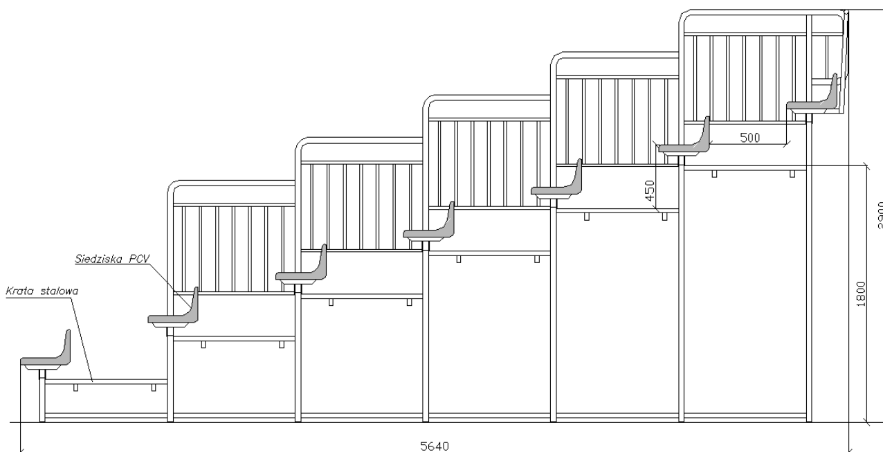
Widok z boku trybuny 7 rzędowej z siedziskami PCV
