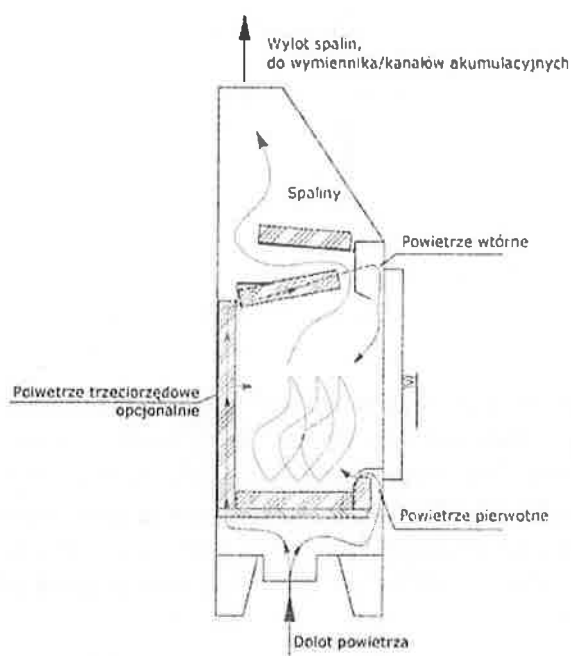
Rys. 1. Dystrybucja powietrza do spalania
